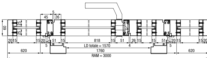
Coupe horizontale de la porte de loft en acier à 2 vantaux avec parties latérales et imposte vitrée
