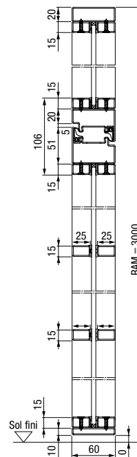
Coupe verticale de la porte de loft en acier à 1 vantail avec parties latérales et imposte vitrée
