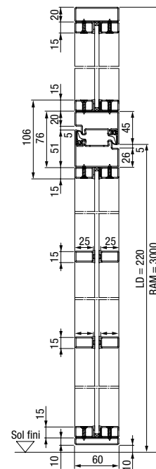
Coupe verticale de la porte de loft en acier à 2 vantaux avec parties latérales et imposte vitrée
