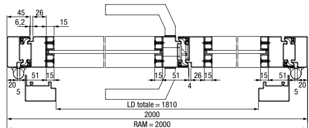
Coupe horizontale de la porte de loft en acier à 2 vantaux
