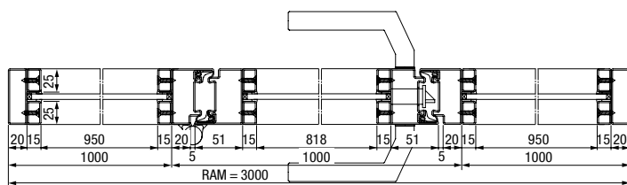
Coupe horizontale de la porte de loft en acier à 1 vantail avec parties latérales et imposte vitrée
