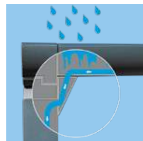
Évacuation de l'eau dans les poteaux
