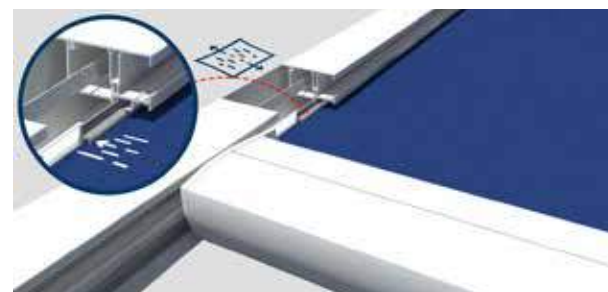
Une toile de toit toujours bien tendue grâce à la tension continue de la technologie de screen ZIP.
